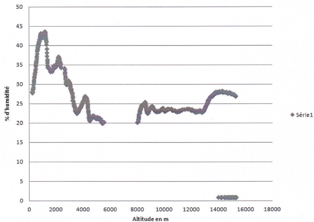
Taux d'humidité dans l'air en fonction de l'altitude
